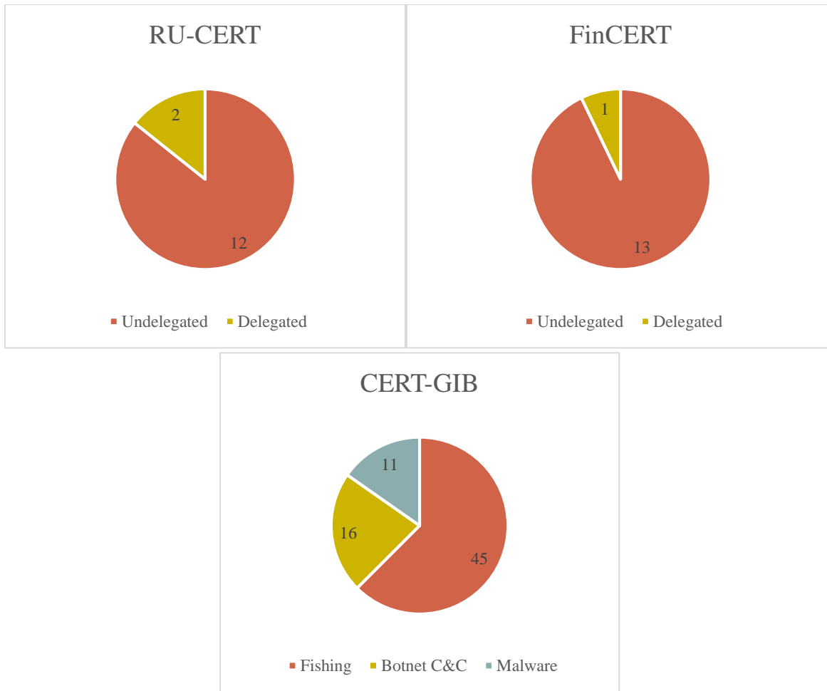
Рис. 7. Инциденты с доменами.
